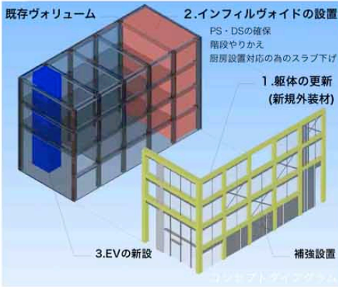
既存ヴォリューム 2.インフィルヴォイドの設置 PS・DSの確保 階段やかえ 厨房設置対応の為のスラブ下げ 1.躯体の更新 (新規外装材) 3.EVの新設 補強設置
